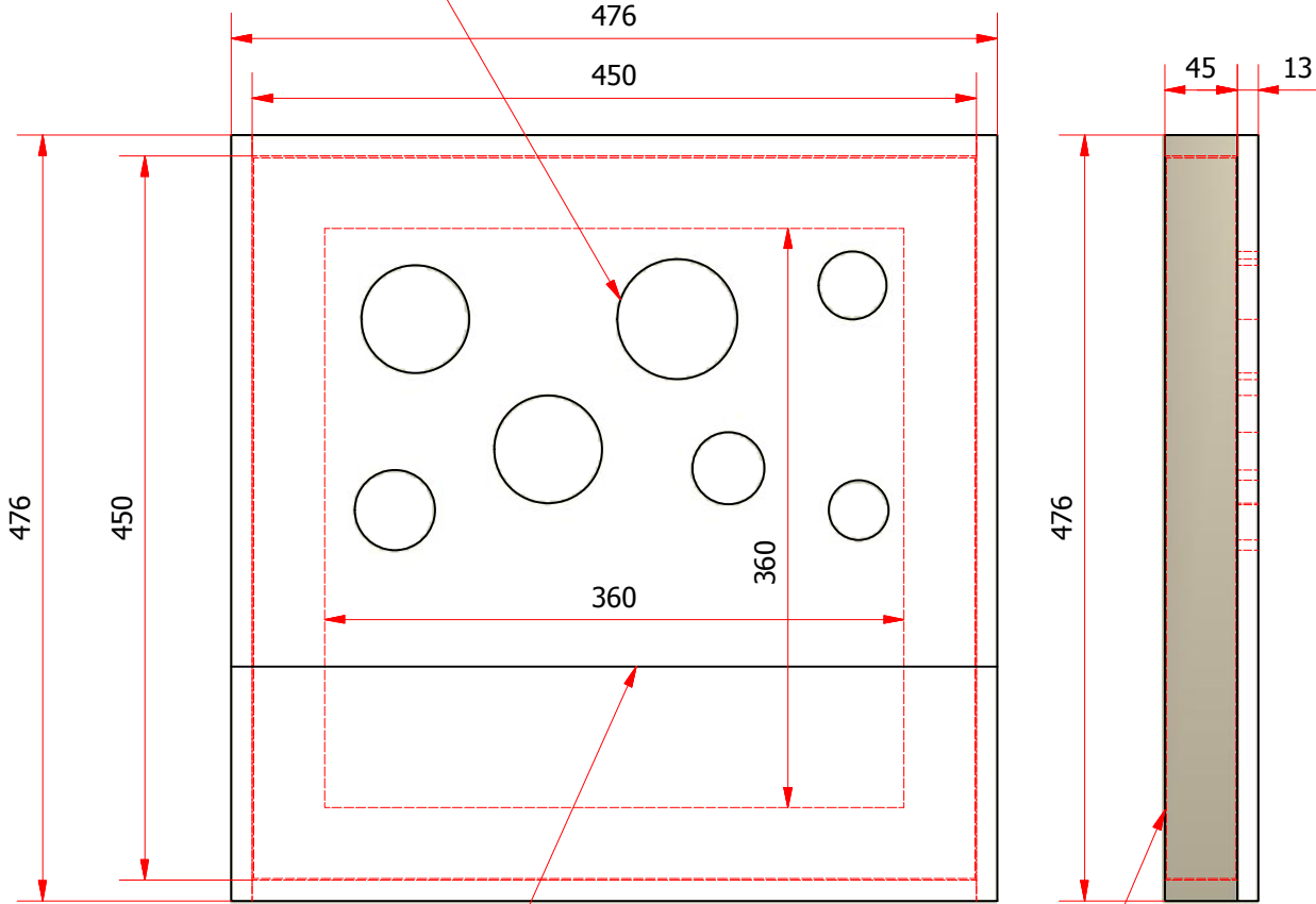
VUE DE FACE ( 1 : 5 )
